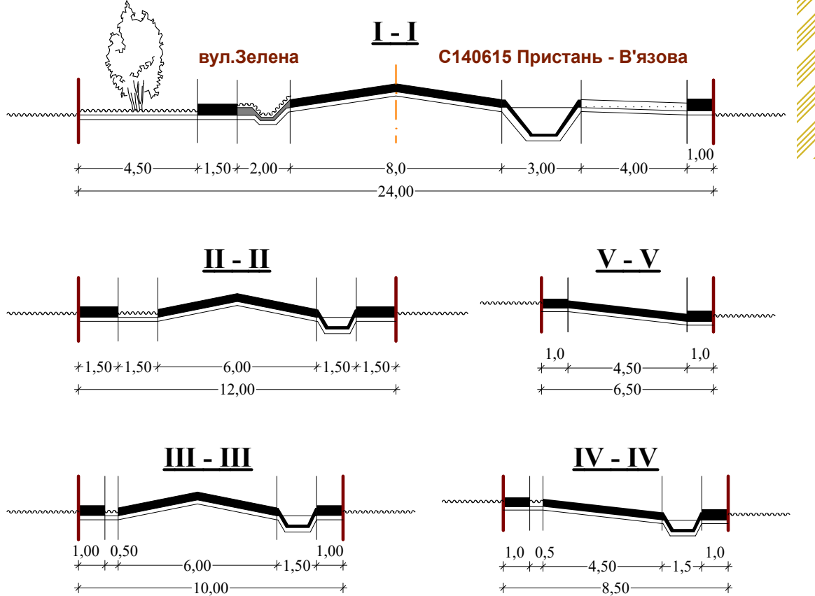
ПОПЕРЕЧНІ ПРОФІЛІ ВУЛИЦЬ ТА ПРОІЗДІВ М 1:200
