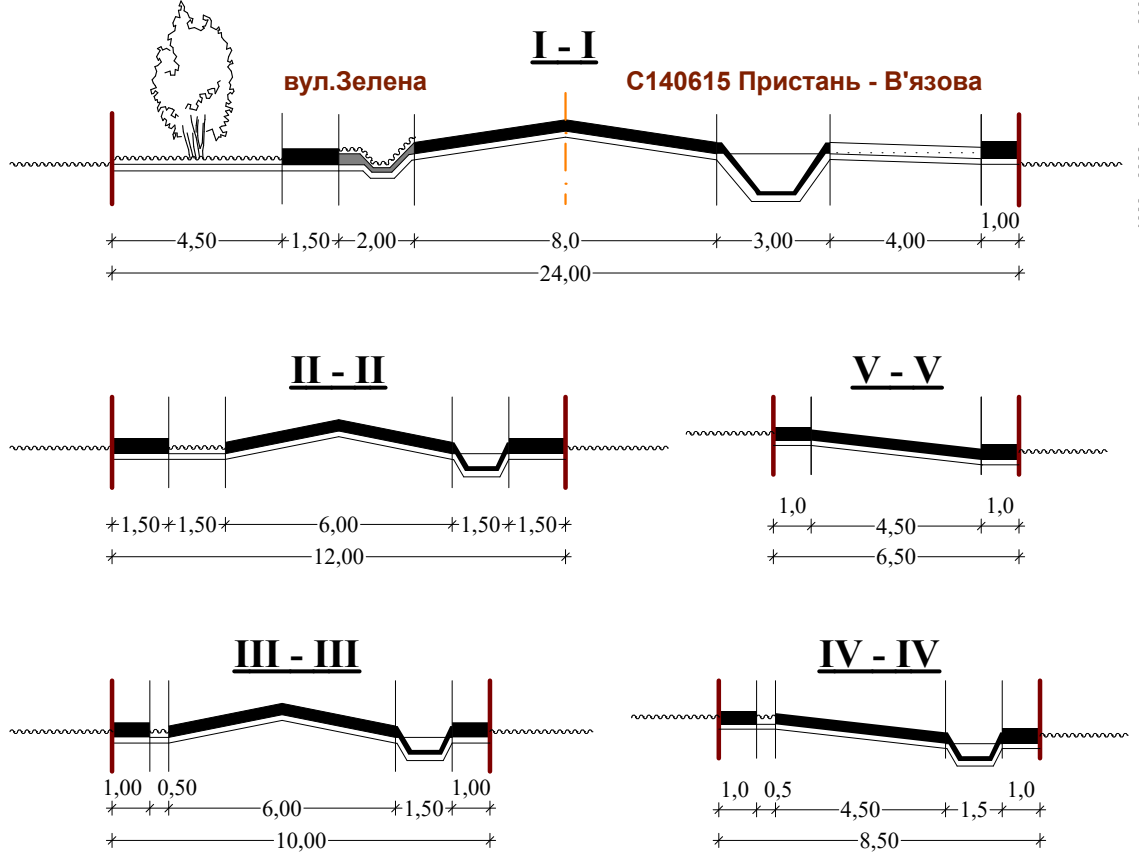
ПОПЕРЕЧНІ ПРОФІЛІ ВУЛИЦЬ ТА ПРОЇЗДІВ М 1:200
