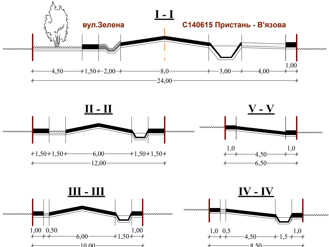
ПОПЕРЕЧНІ ПРОФІЛІ ВУЛИЦЬ ТА ПРОІЗДІВ М 1:200
